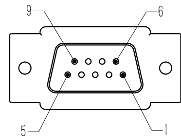
DB-9插头示意图
