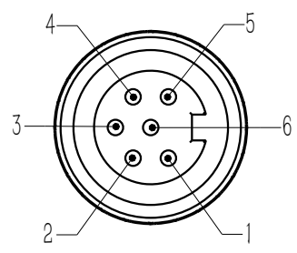
6Pin航插示意图
